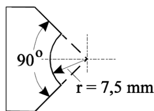
NOSE TEMPLATE
